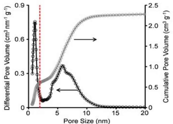
Meso-makroporöse Kohlenstoffe. Linkes Bild: SEM-Aufnahme; rechtes Bild: Porengrößenverteilung basierend auf \text{N}_2 -Physisorption.
