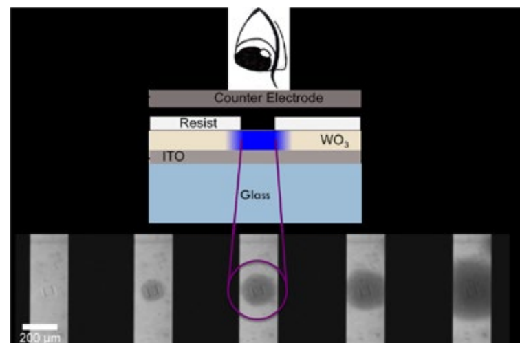
Schematische Darstellung der Versuchsanordnung zur ortsaufgelösten Untersuchung lateraler Transportprozesse. Unten: Optische Mikroskopbilder der Probenoberfläche, eine rechteckige Aussparung ist erkennbar, durch die Ionen lokal in die Schicht eingebracht werden. Von links nach rechts zeigt sich die sukzessive Einfärbung der Schicht aufgrund seitlicher Ionenwanderung.
