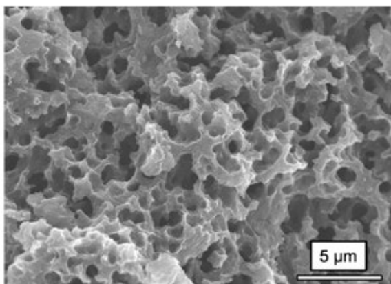
Meso-makroporöse Kohlenstoffe. Linkes Bild: SEM-Aufnahme; rechtes Bild: Porengrößenverteilung basierend auf \text{N}_2 -Physisorption.
